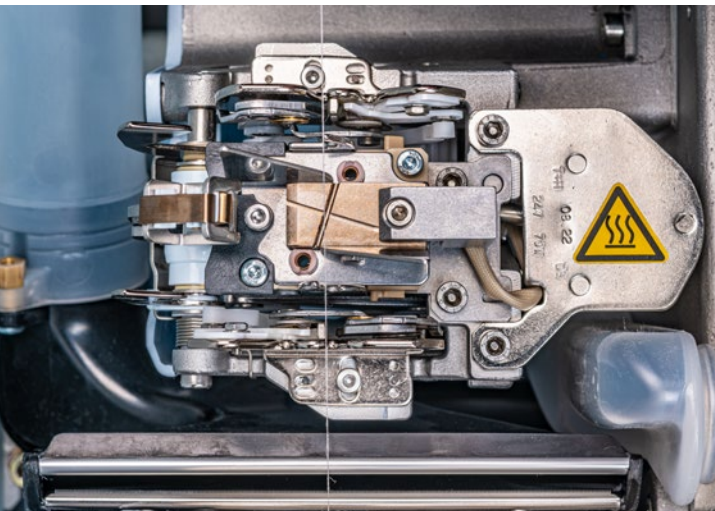
Thermosplicer热捻接器
