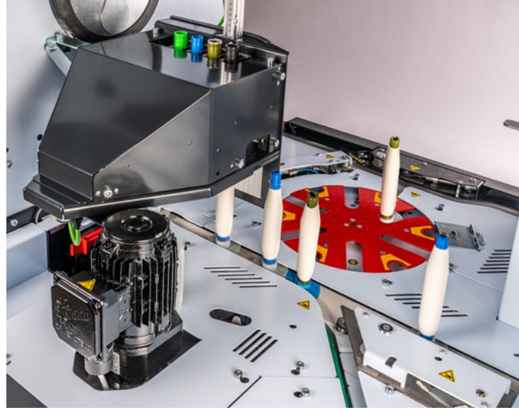
配备新型管色检查功能的自动络筒机Autoconer X6
