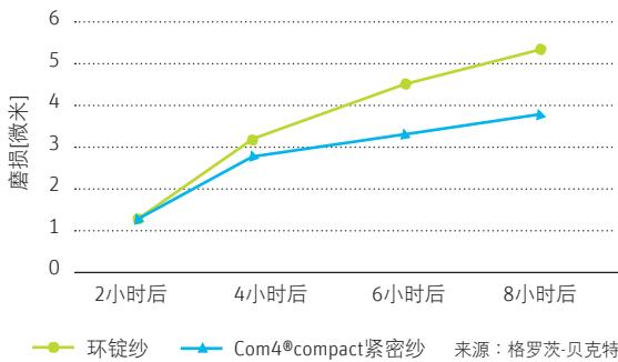
针织机的织针磨损
