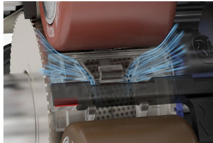
采用气流导向控制元件，减少了空气流量
