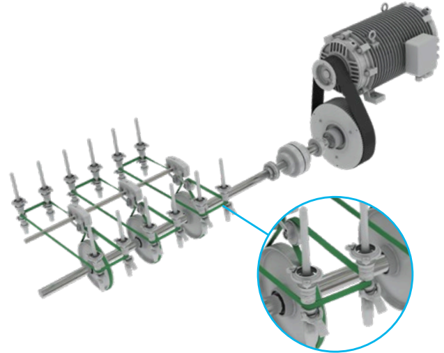
90度缠绕有助于实现出色的能源传递，降低能耗
