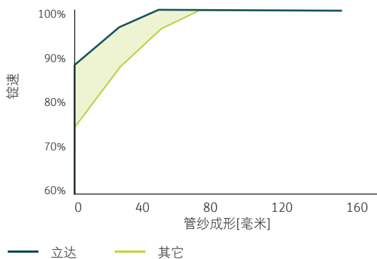
在相同的最高锭速下，产量提升可达2%
