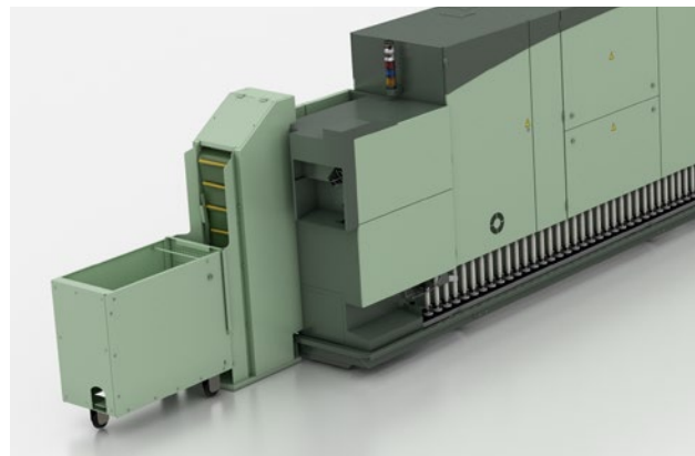
WILDload系统：纱管被逐个拣出，经过对齐后喂入纱管装载装置ROBOload中。
