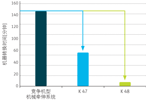
使用全电子(K 48)系统的额外优势
