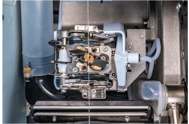
自动络筒机Autoconer X6带有喷湿捻接器
