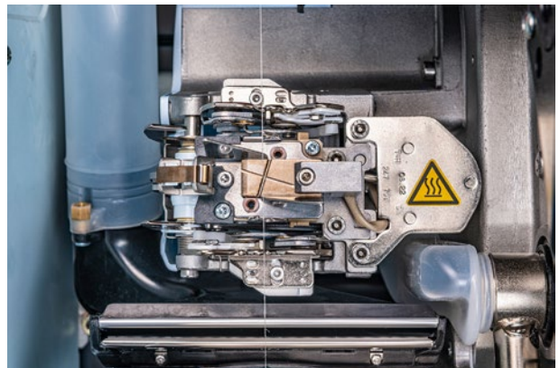
自动络筒机Autoconer X6带有Thermosplicer热捻接器
